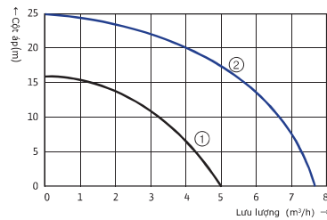
Đường đặc tính bơm
